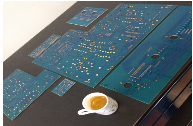
Vue ds circuits: Un ensemble de 8 circuits imprimés de 4 à 8 couches à double épaisseur de cuivre (70uM). Avec des composants des deux cotés.
