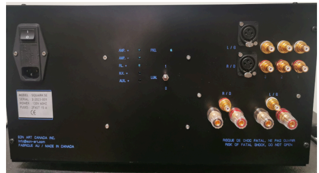
Vue de l'arrière: Connectique de haute qualité de chez Neutrik et Supra
